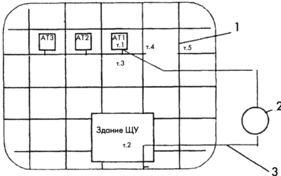
Рис. П2.1. Схема прокладки магистралей ЗУ:
