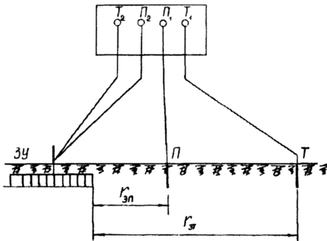
Рис. 2. Принципиальная схема измерений сопротивления ЗУ:
