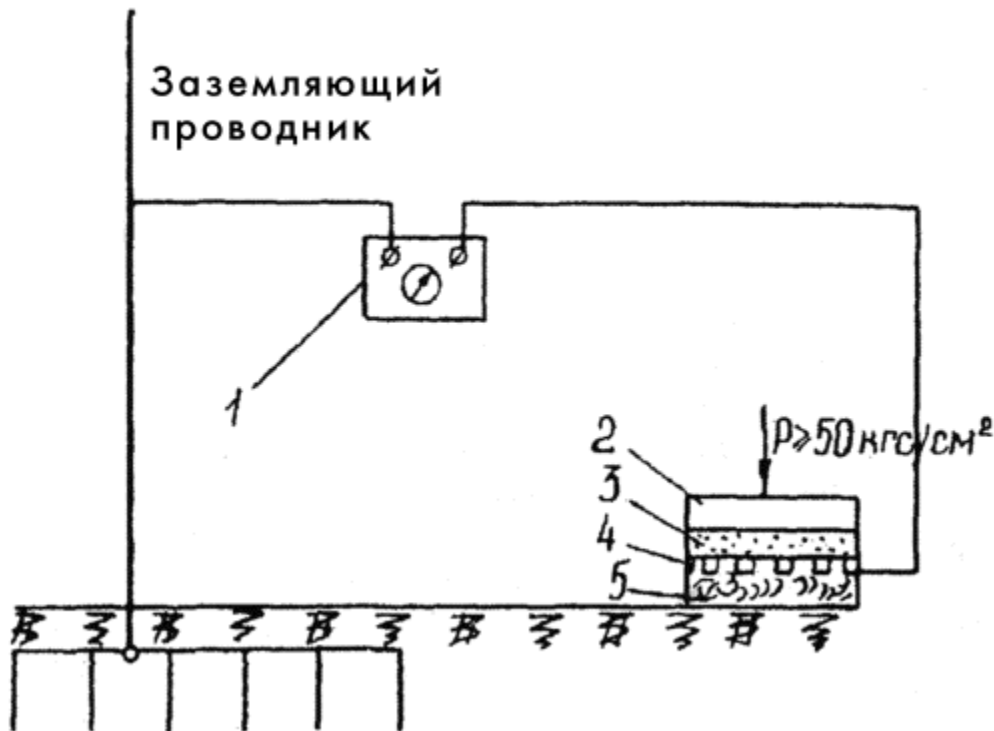
Рис. 9. Схема измерения сопротивления основания:
