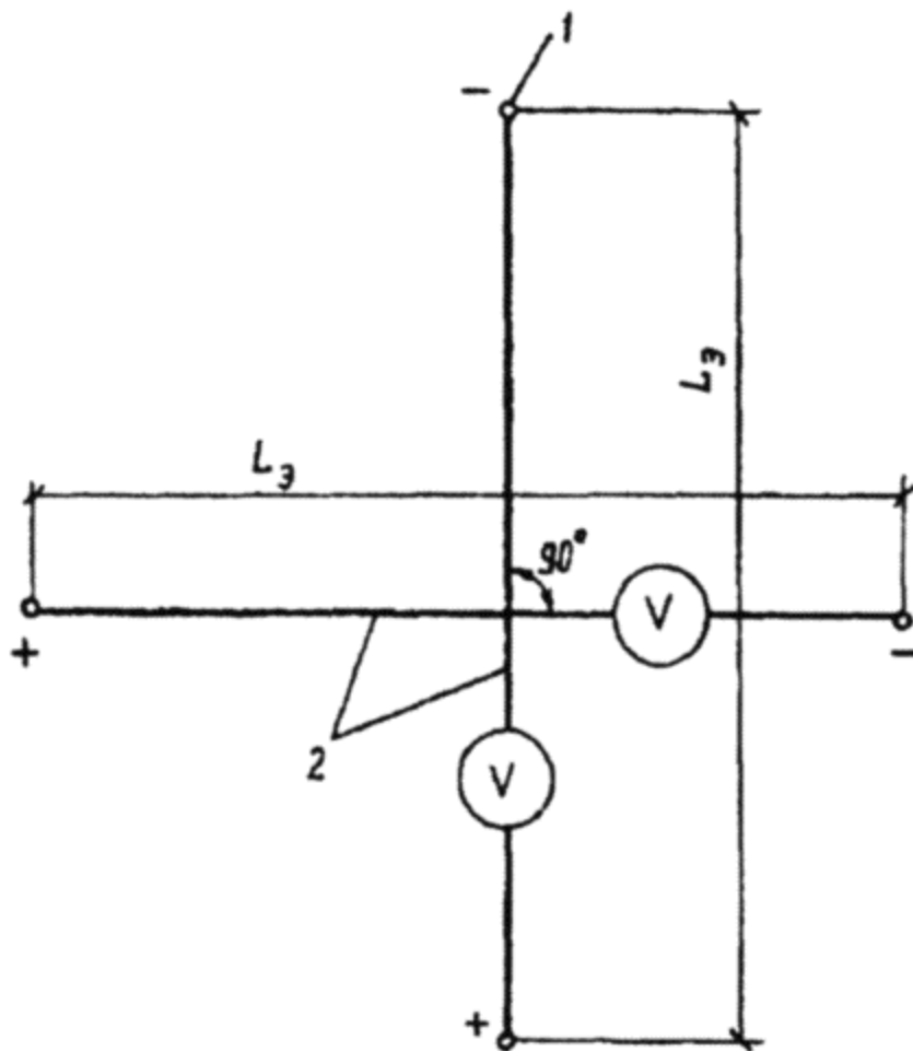
Рис. ПЗ.3. Схема измерений для обнаружения блуждающих токов в земле:
