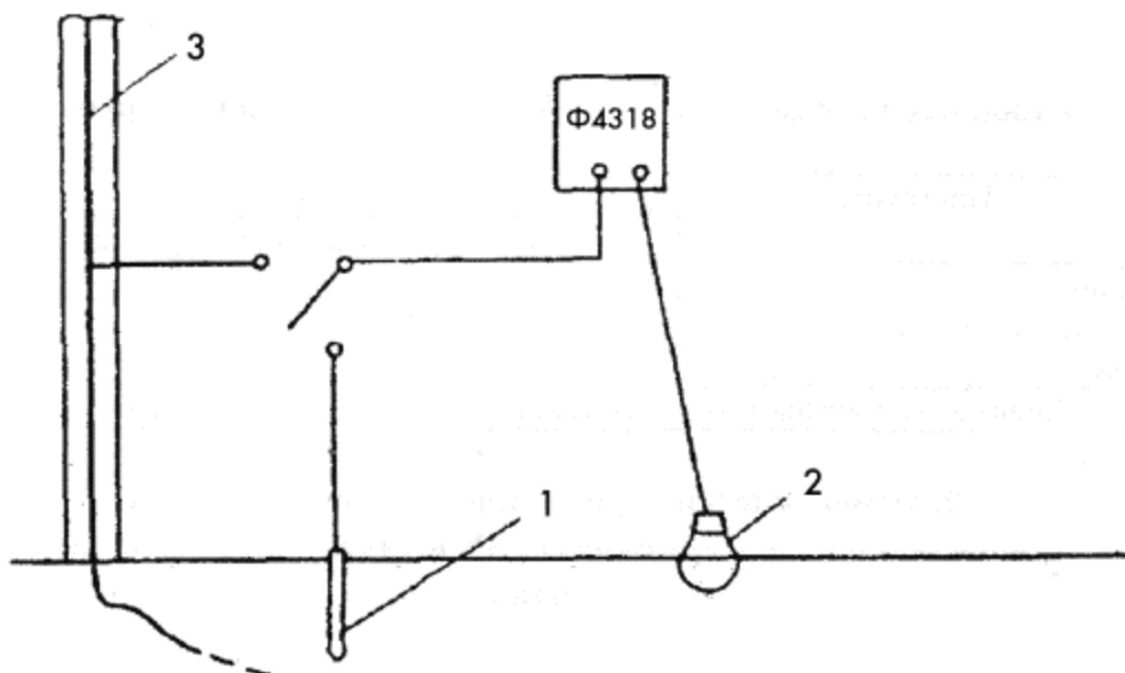
Рис. ПЗ.1. Схема измерения электрохимического окислительно-восстановительного потенциала:
