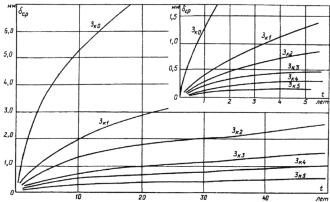
Рис. ПЗ.2. Рост средней глубины фунтовой коррозии стали
