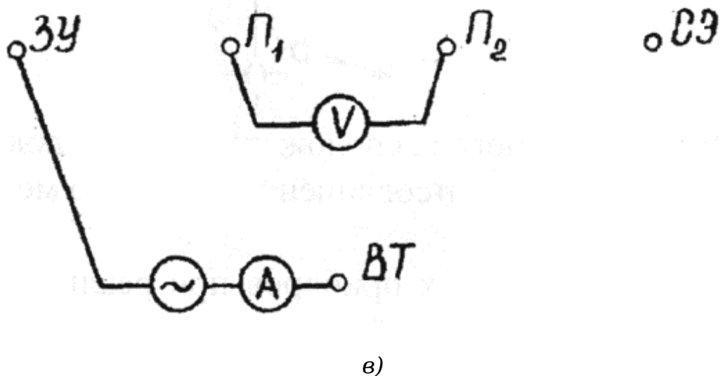
Рис. 5. Схемы трех последовательно используемых вариантов включения измерительных приборов при измерениях по методу СибНИИЭ (см. рис. 4 )
