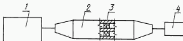
1 — панорамный измеритель модуля коэффициента передачи и отражения; 2 — коаксиальный расширитель; 3 — образец ПЭВ; 4 — согласованная нагрузка
