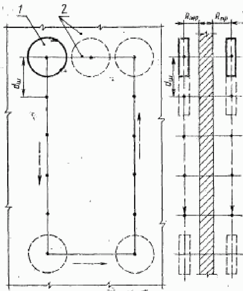
1 — рамочная антенна; 2 — волотно дверного проема
