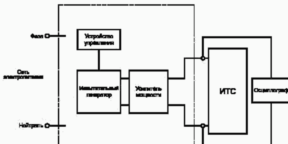
Рисунок Б.1б — Схема устройства для испытаний при воздействии провалов, прерываний, выбросов и постепенных изменений напряжения с использованием усилителя мощности
