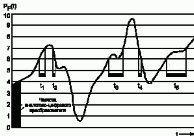
Рисунок 2а — Уровень фликера как функция времени
